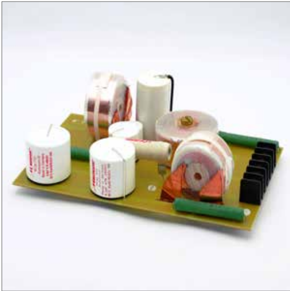
MCap分频器版本《C》
