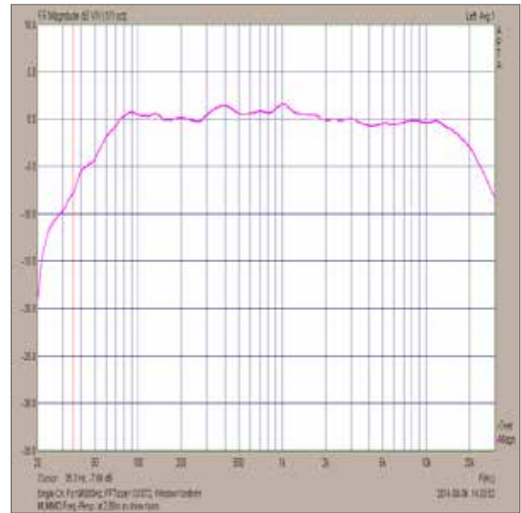
MA30的频率响应
