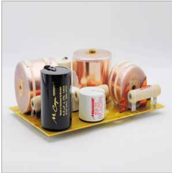
MCap分频器版本《B》
